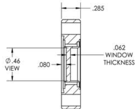
SECTION A-A SCALE 1.5 : 1
