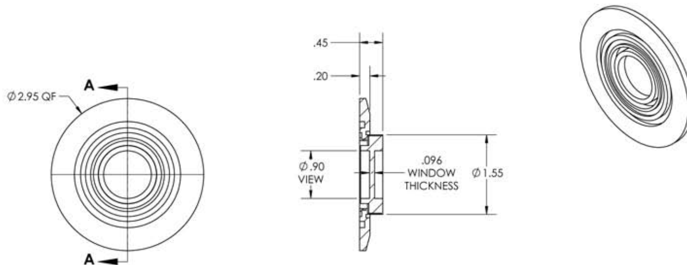
SECTION A-A SCALE 1 : 1.5
